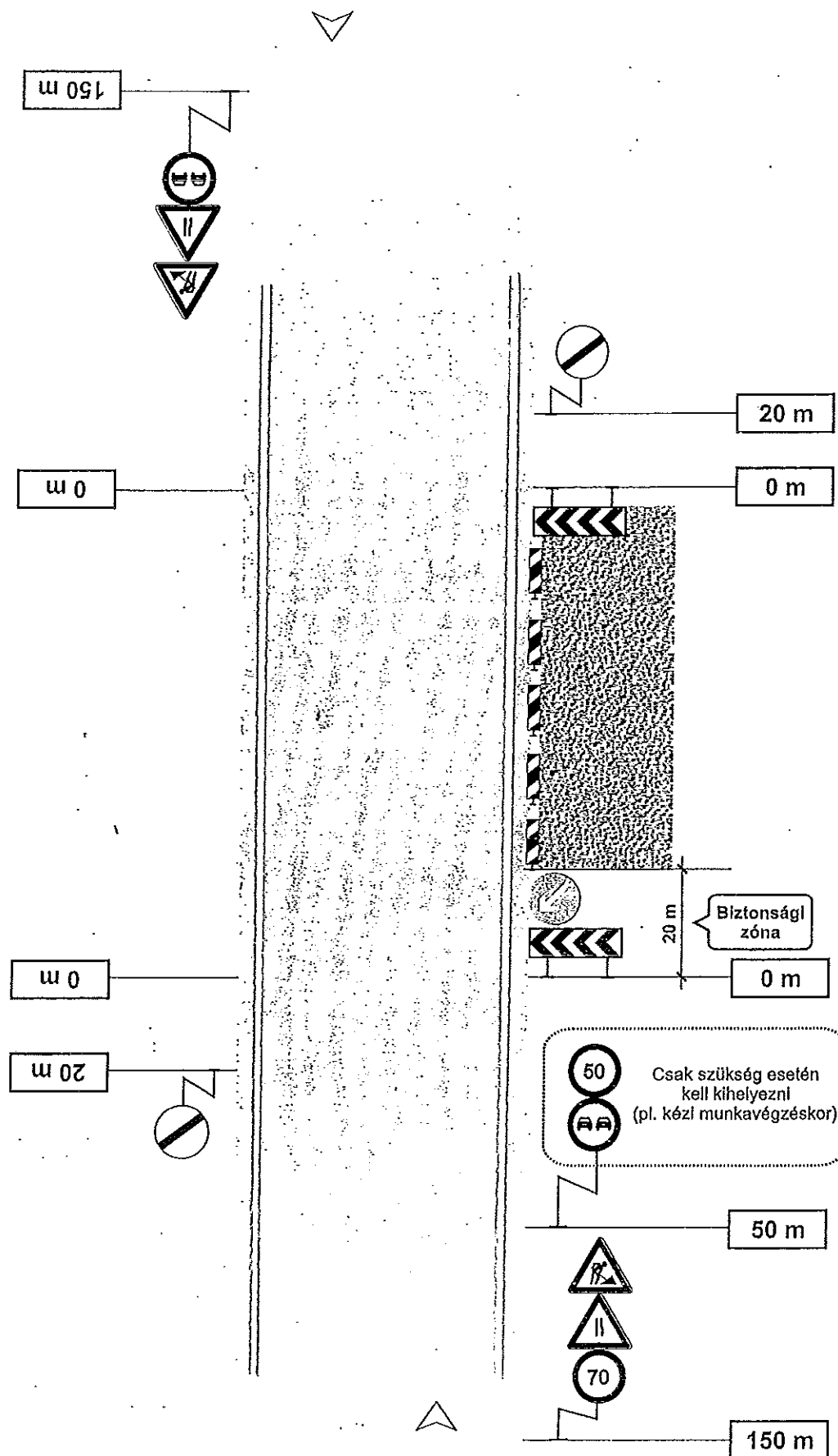
5.1.2. ábra – Útpadkán lévő munkaterület (az úttest és a munkaterület szintkülönbsége 5 centiméternél kisebb)
